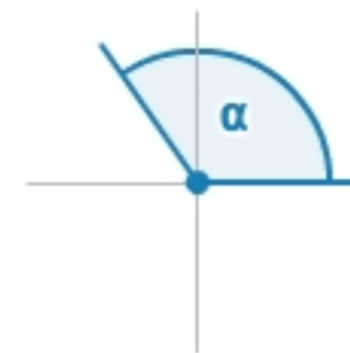
stumpfer Winkel 90^\circ < \alpha < 180^\circ
