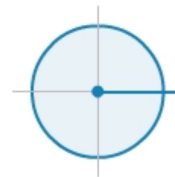
voller Winkel 360^\circ
