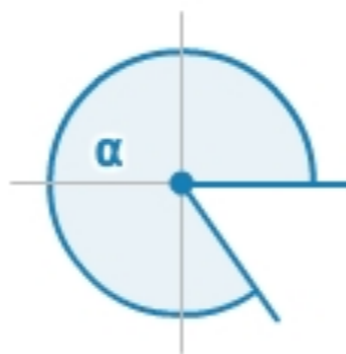
überstumpfer Winkel 180^\circ < \alpha < 360^\circ
